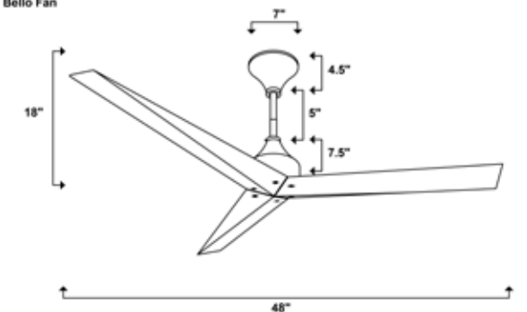
Size Chart Bello Fan
