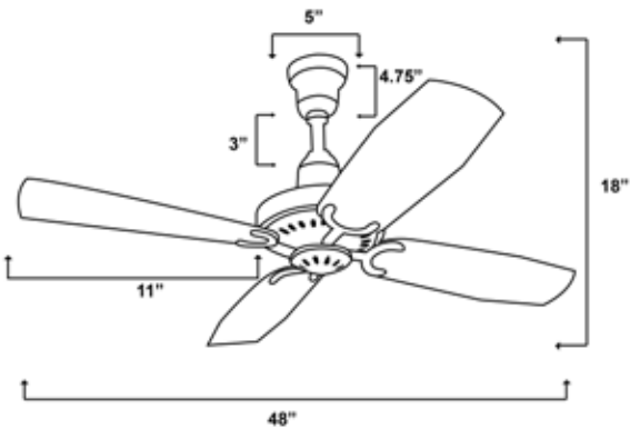
Size Chart Era fan
