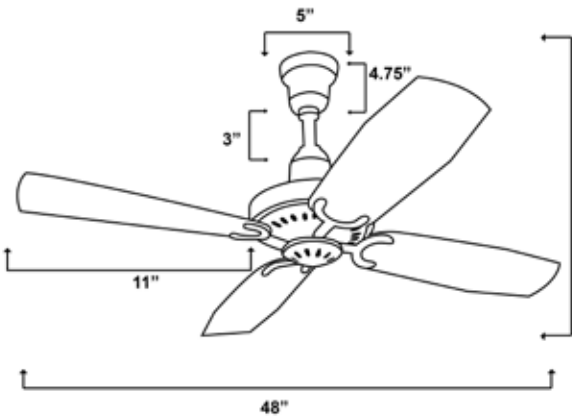
Size Chart Era fan
