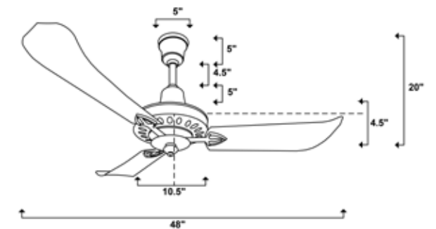
Size Chart Eminent Fan
