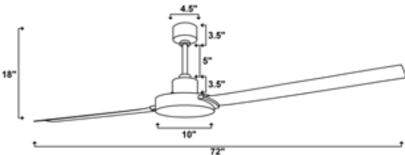
Size Chart Helious 2-Blade Fan
