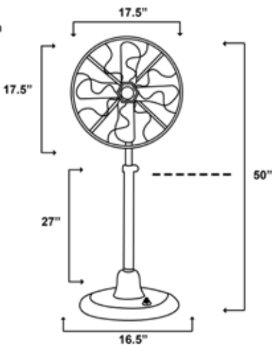
Size Chart Pedestal metal fan
